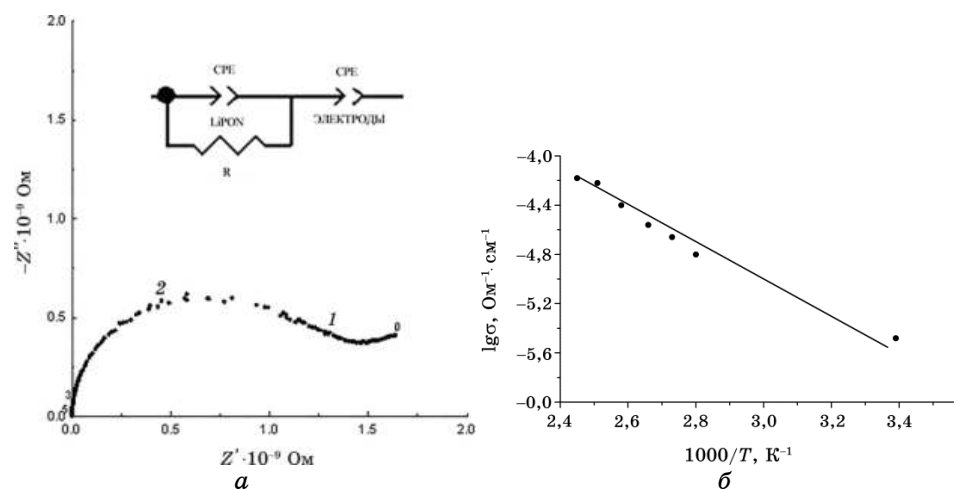
Рис. 3. а — диаграмма комплексного импеданса в координатах Найквиста плёнки LiPON при 20^\circ\text{C} (цифры над кривой — логарифм частоты); б — температурная зависимость проводимости плёнки LiPON.
